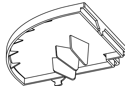
下方斜視図
